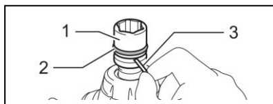
1-ударная головка 2-Уплотнительное кольцо 3-Штифт
