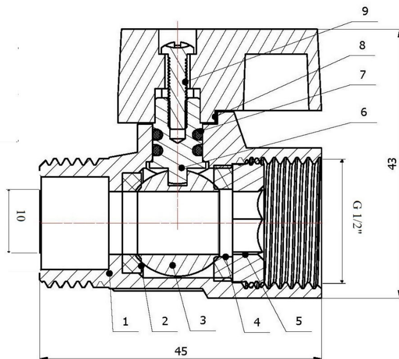
Рис.2. Габариты крана 1/2"
