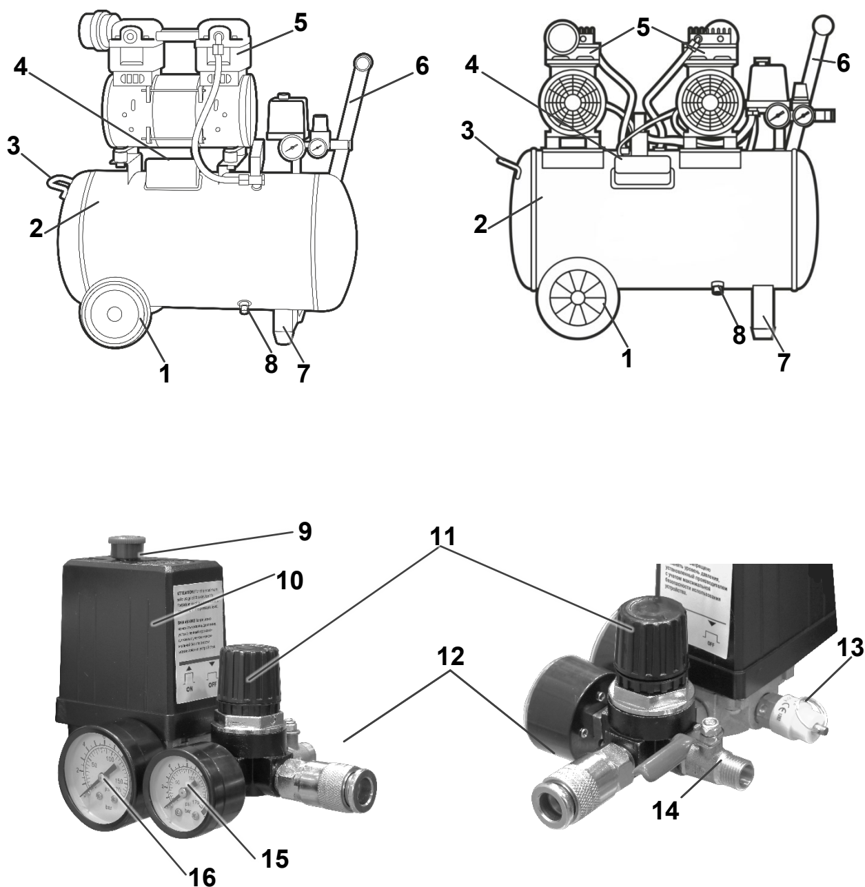
Figure 2 – Diagram of AE-10-OF1 / AE-25-OF1 / AE-50-OF1 Compressors 2-сурет – AE-10-OF1 / AE-25-OF1 / AE-50-OF1 компрессорларының схемасы Рисунок 2 – Схема компрессора AE-10-OF1 / AE-25-OF1 / AE-50-OF1
