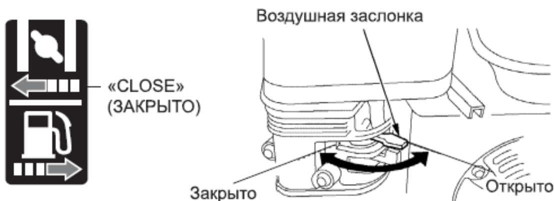
Рисунок 14 – Воздушная заслонка
