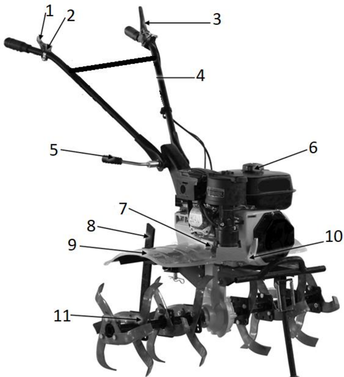
Рисунок 1 – Основные части и узлы культиватора
