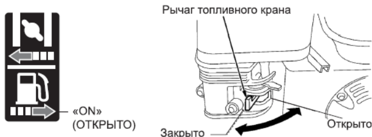
Рисунок 9 – Топливный кран
