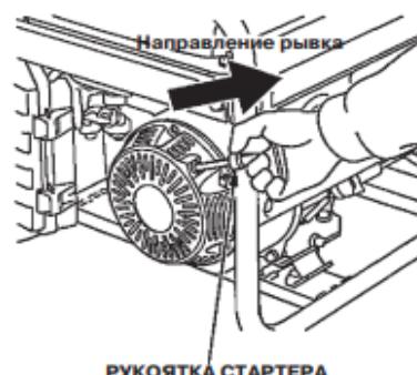
РУКОЯТКА СТАРТЕРА
